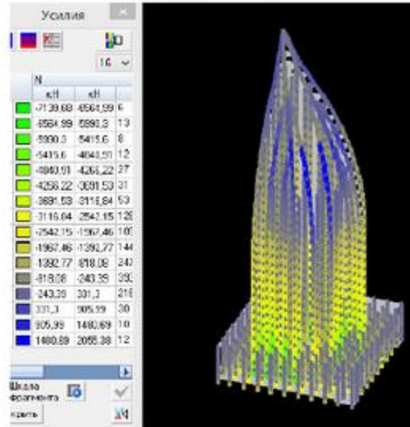
Изоляция усилий N в колоннах
