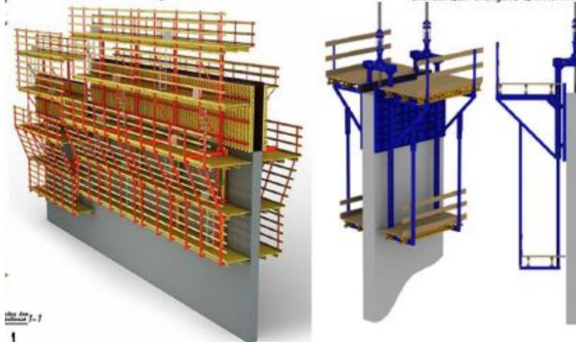
Самостоятельная опалубка Peri ACS
